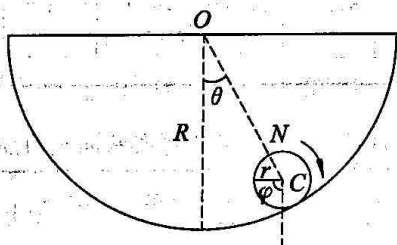
图 1 小球在碗内做纯滚动
