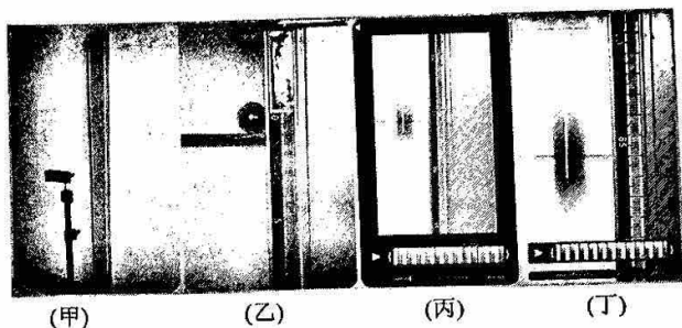
图 5 实验过程中的几个关键步骤
