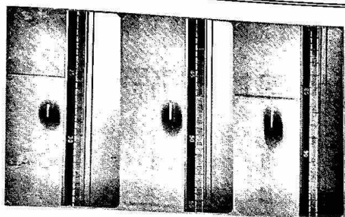
图 4 每秒 240 帧模式下钢球不同位置的分帧图片
